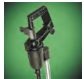
Mini 360 border sprinkler on 1m metal rod
